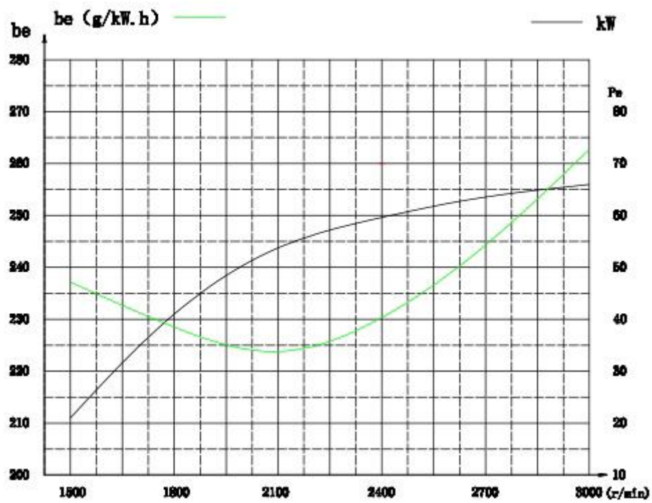
4BD-G 3000转特性曲线图
